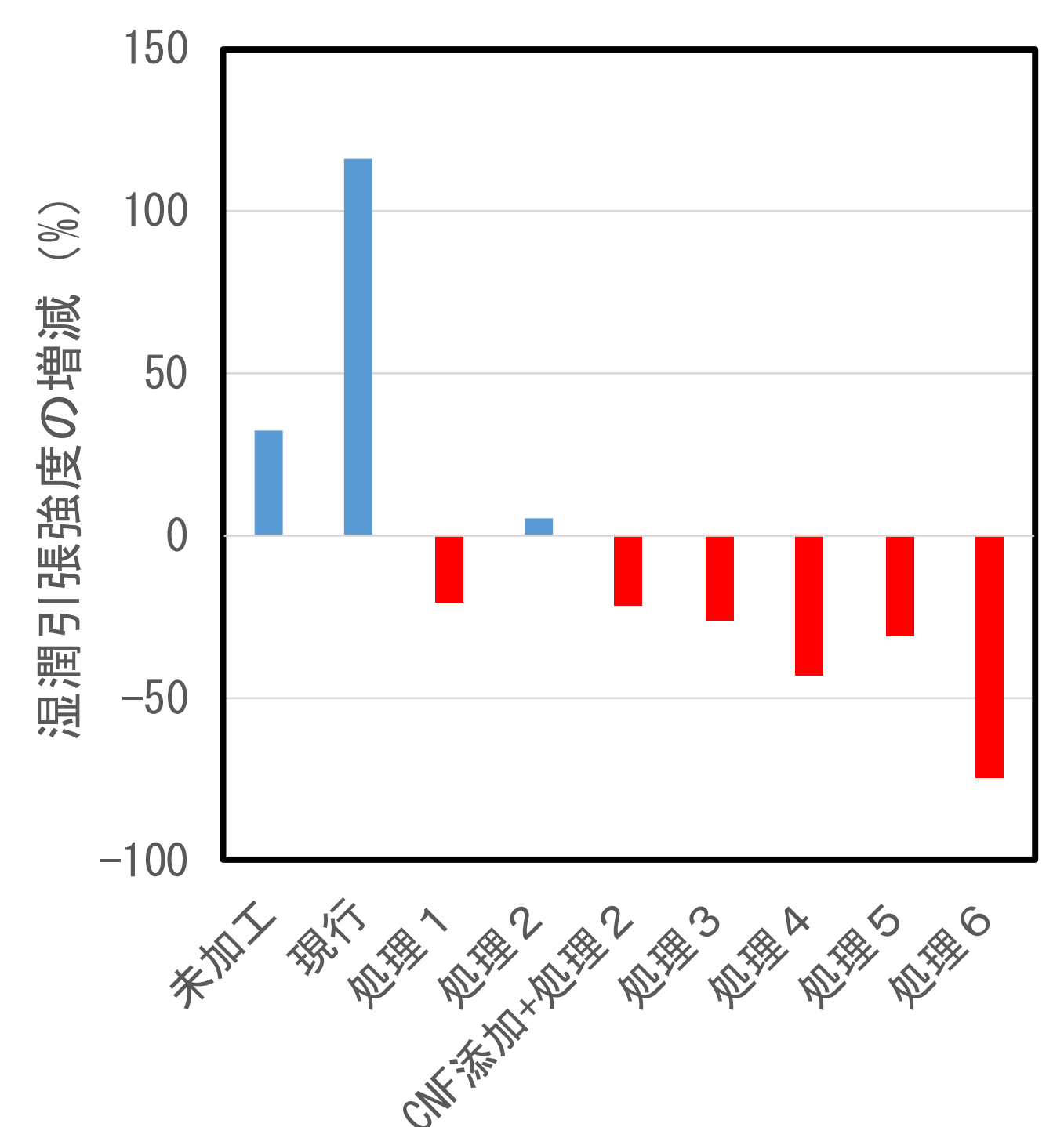
図2 乾湿試験前後の湿潤引張強度の増減
