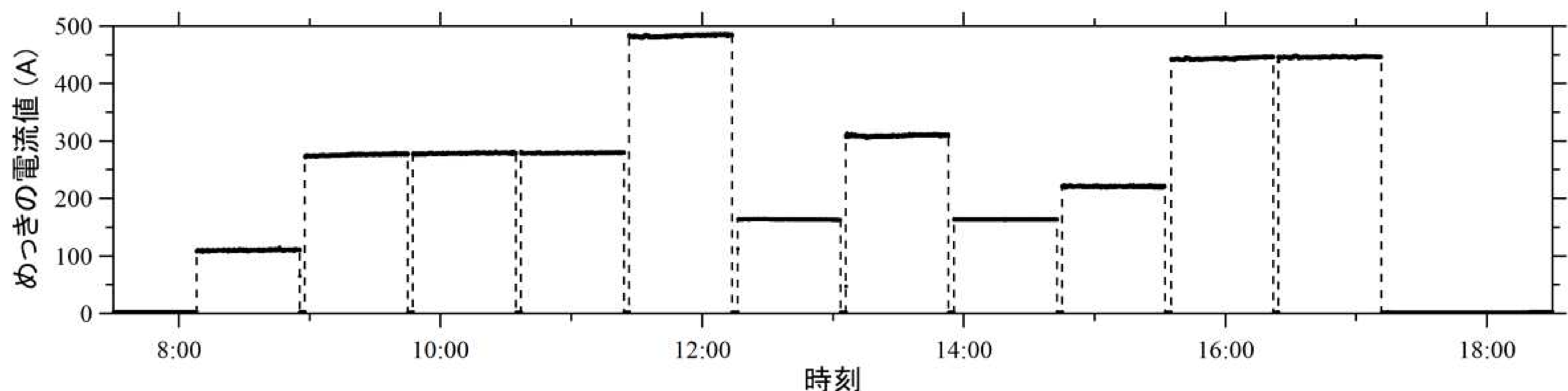
図1 工場におけるバレルめっき整流器の直流電流値ログの例，データは1秒おきに取得
